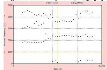
Fig 2.1, traiectorie formanți S 4 [find]
